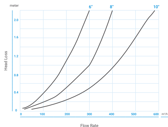
NR-010 6" - 10"
