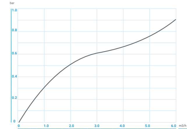
1" PRV
