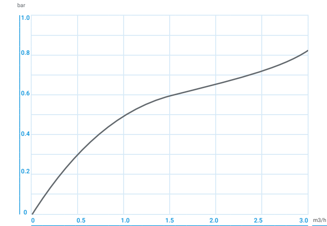
3/4" PRV
