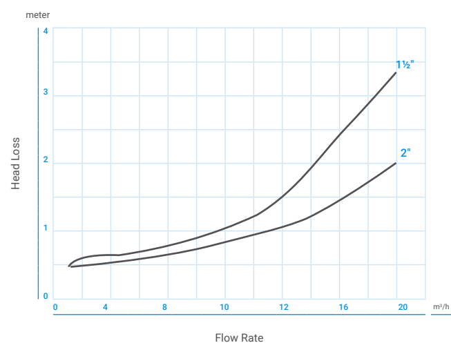
NR-010 1½", 2"
