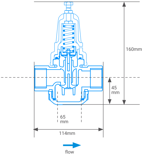
1" PRV
