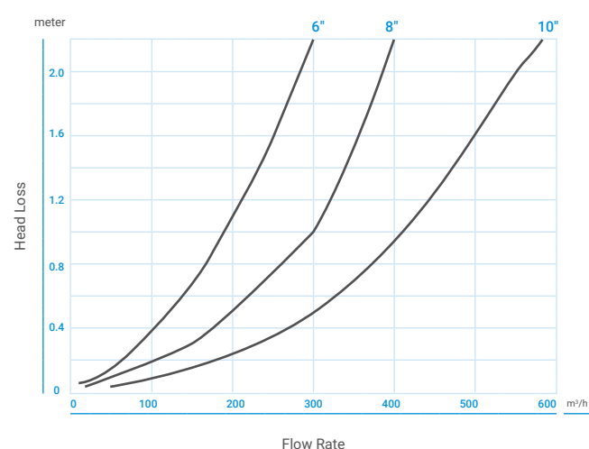
NR-010 6" - 10"
