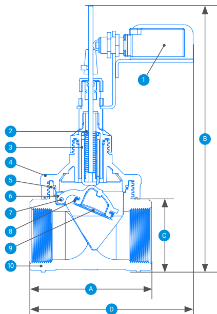
NR-010 1½", 2"
